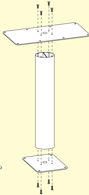
Esempio di blocchiera MODULAR assemblata con mantello e piantana
