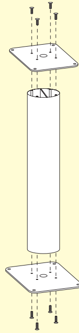
Piantana con piastra piccola. Support column with small plate.
