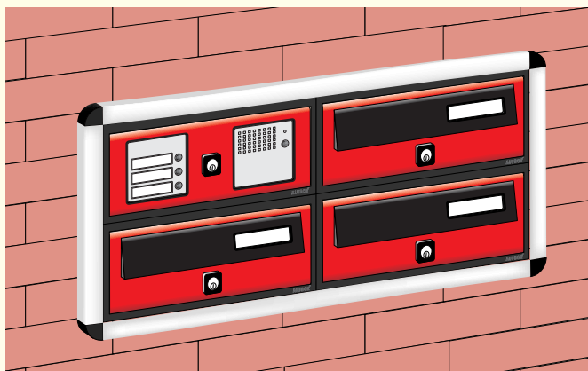
Composizione da incasso con cornice coprifuga Recess mounting set with cover frame
