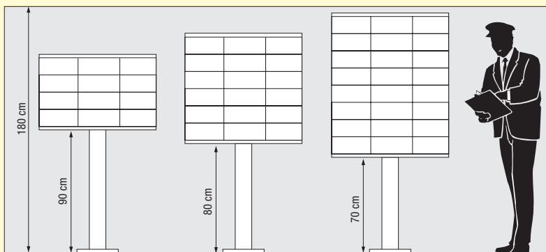
Piantana con piastra grande. Support column with big plate.
