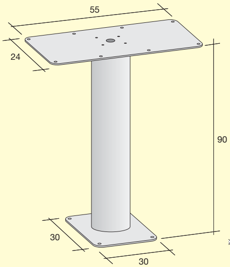
Piantana con piastra grande. Support column with big plate.
